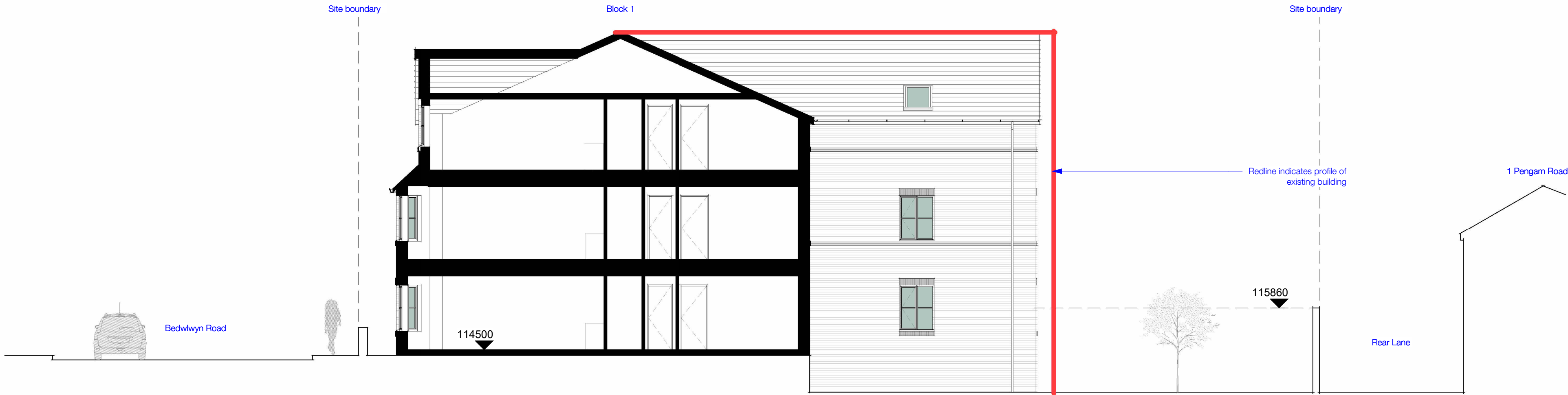
Site section 1 1 : 100
